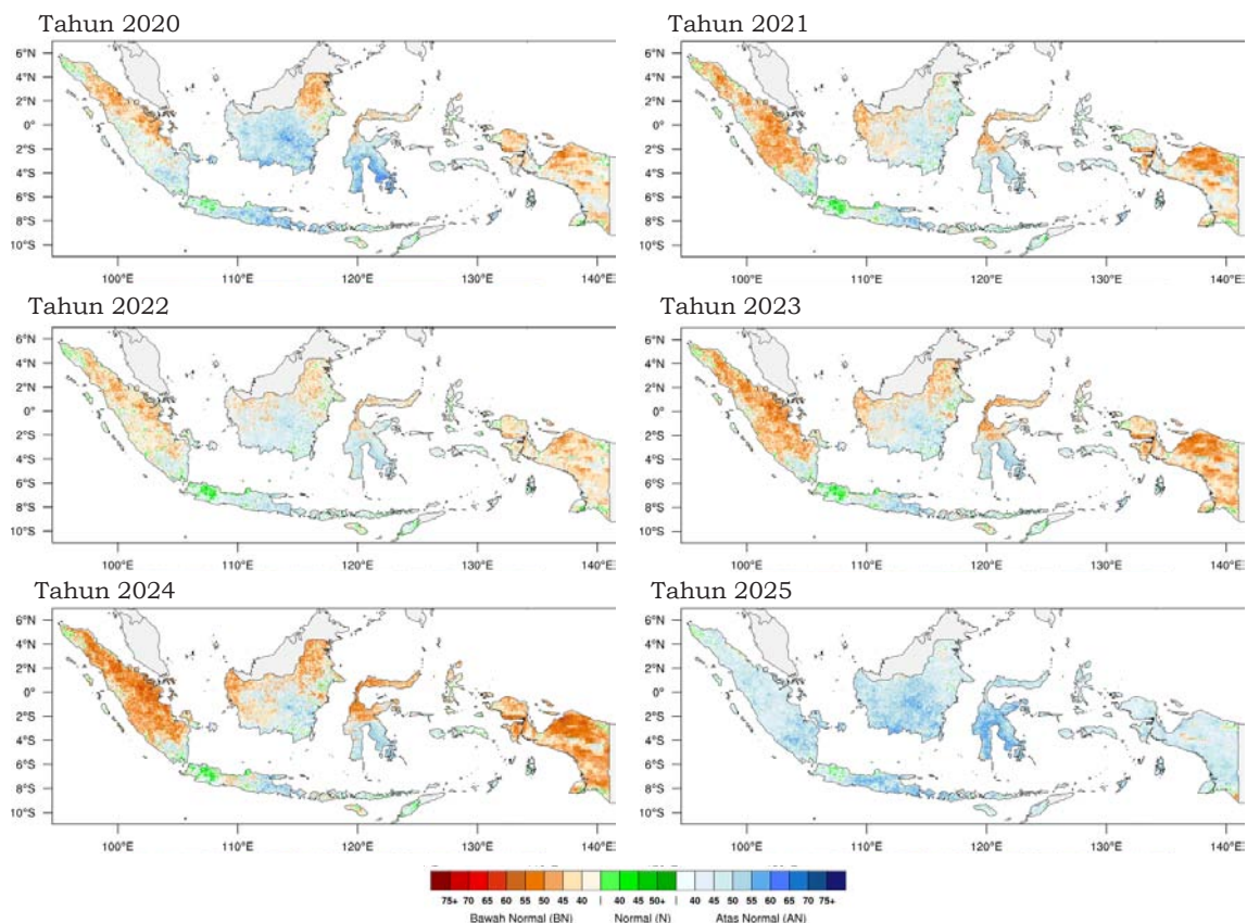
Gambar 7.8 Prediksi Peluang Kejadian Iklim Ekstrem Basah Tahun 2020-2025
