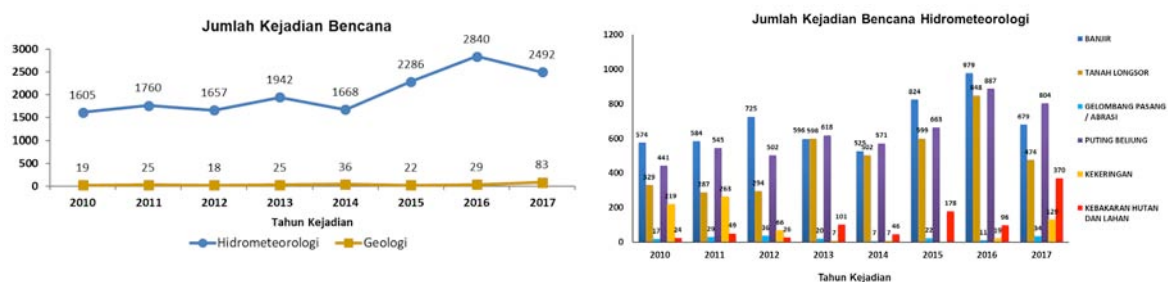
Gambar 7.2 Grafik Perbandingan Bencana dan Jumlah Kejadian Bencana Hidrometeorologi
