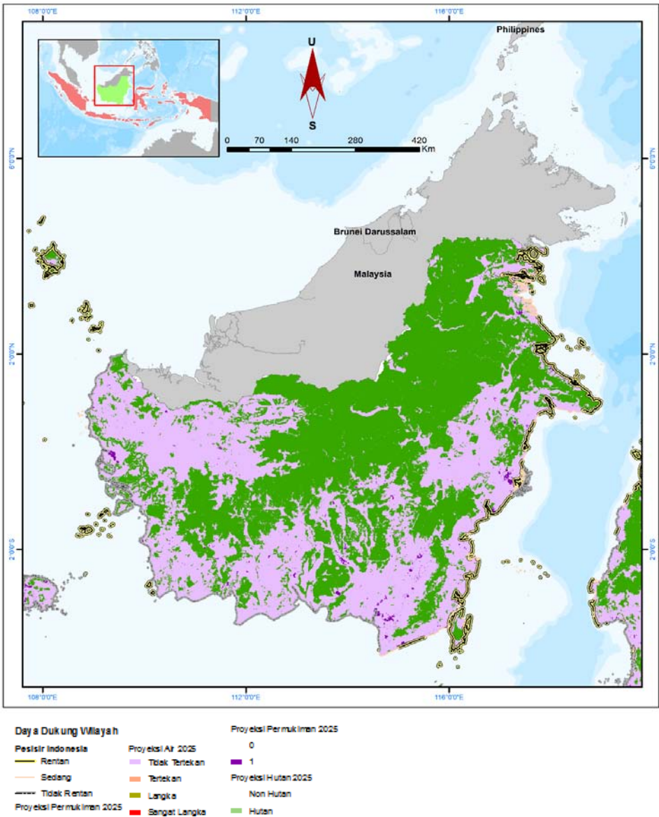
Gambar 5.6. Peta Proyeksi Daya Dukung Lingkungan Wilayah Kalimantan Tahun 2025
