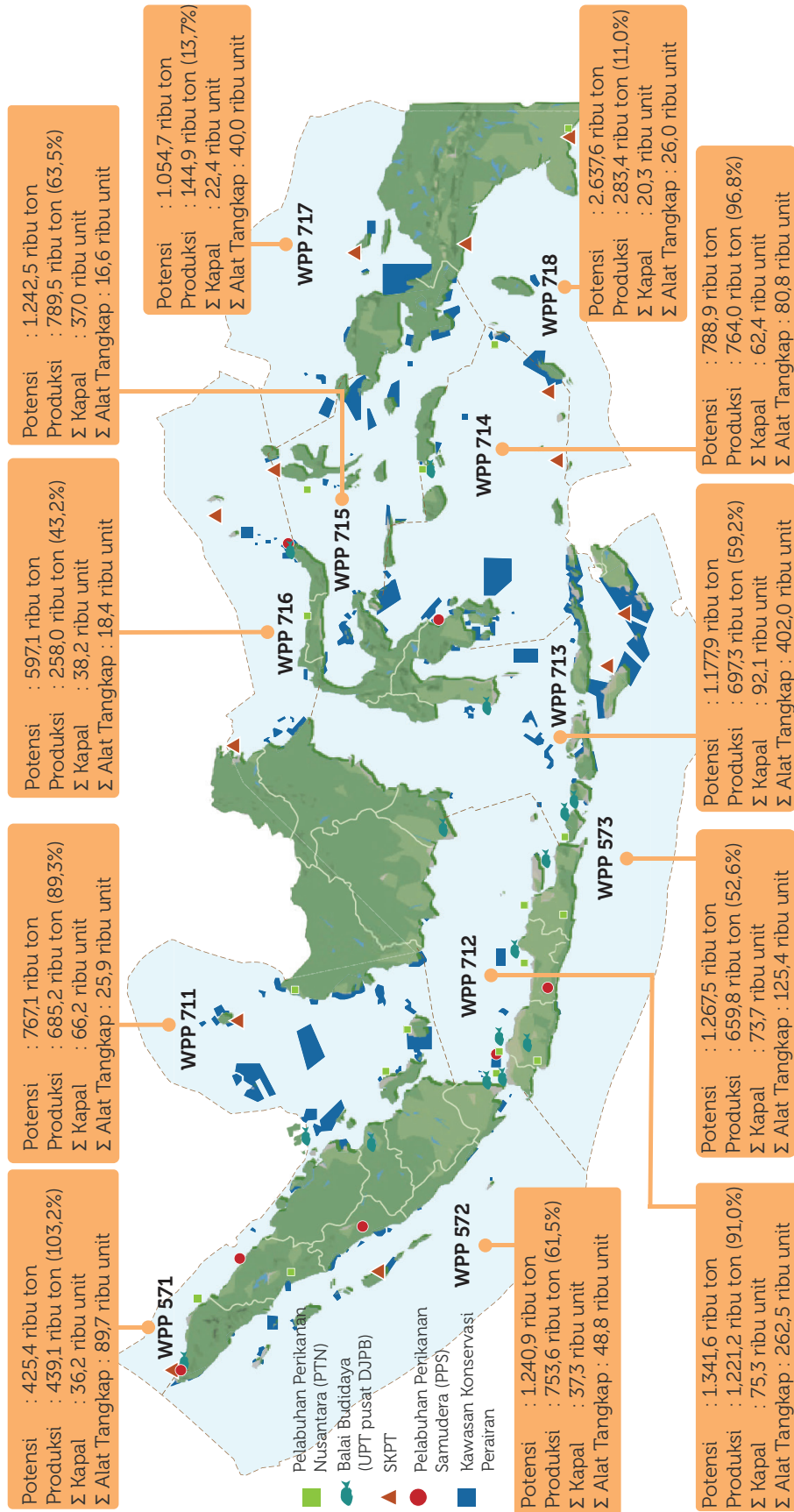
Gambar 3.7 Persebaran Wilayah Pengelolaan Perikanan (WPP)
