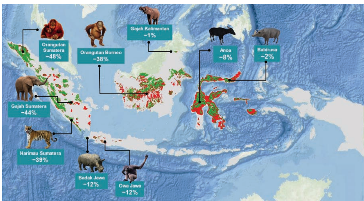
Gambar 1.14 Proyeksi Penyusutan Tutupan Hutan pada Habitat Beberapa Spesies Kunci Tahun 2000-2045
