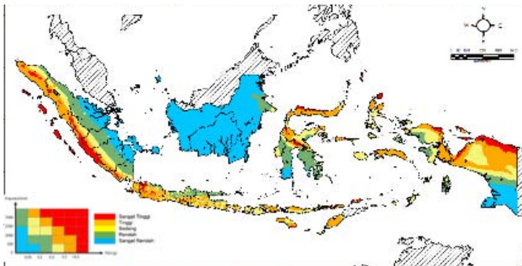
Gambar 7.4 Paparan dan Kerentanan terhadap Bahaya Bencana Gempa bumi dan Sesar Aktif
